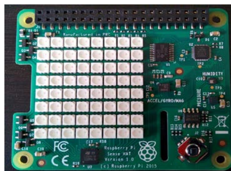
図3 SenseHAT の基板
