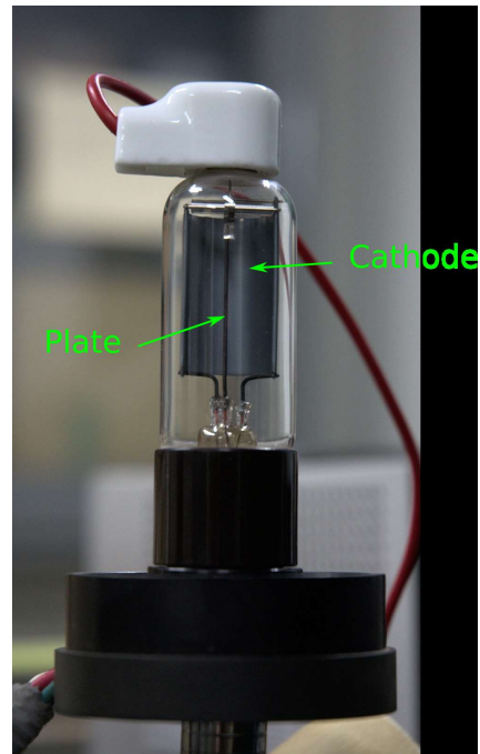
図2 光電管
