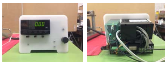
図3 制御盤（表、裏）
