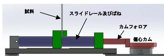
図2 加振機構
